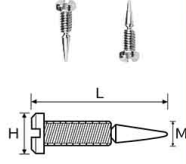
自断螺丝 Self Breaking Screw
