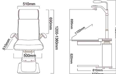
电动升降，可以90°旋转。 Electric power chair 90° rotating.
